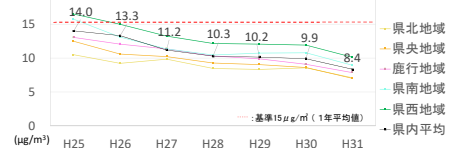
図3 県内の年平均値の推移
