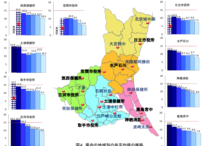
図4 県内の地域別の年平均値の推移
