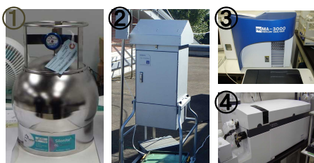
図2 試料採取及び分析用装置の例
