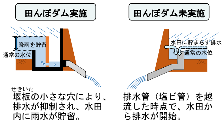
田んぼダム用の落水柵
