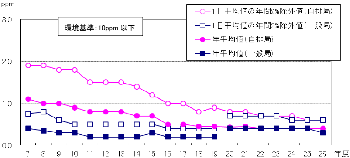
図 2 一酸化炭素濃度の経年変化
