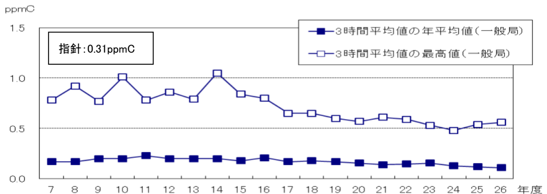
図6 非メタン炭化水素濃度（午前 6 時～9 時における 3 時間平均値）の経年変化
