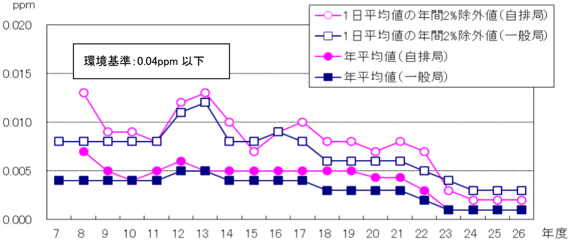
図 1 二酸化いおう濃度の経年変化
