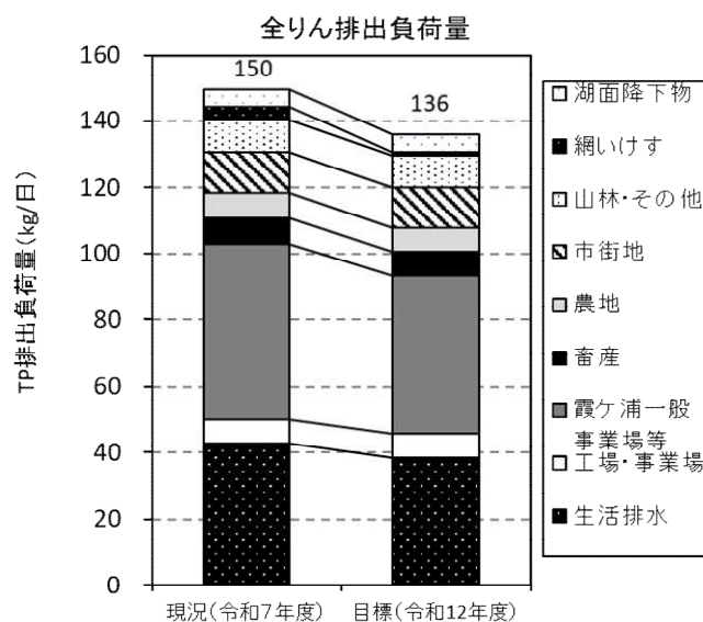
図 15 北浦における排出負荷量（現況及び目標）
