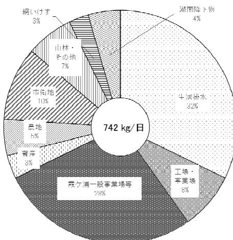
霞ヶ浦におけるTP排出負荷量(令和7年度)
