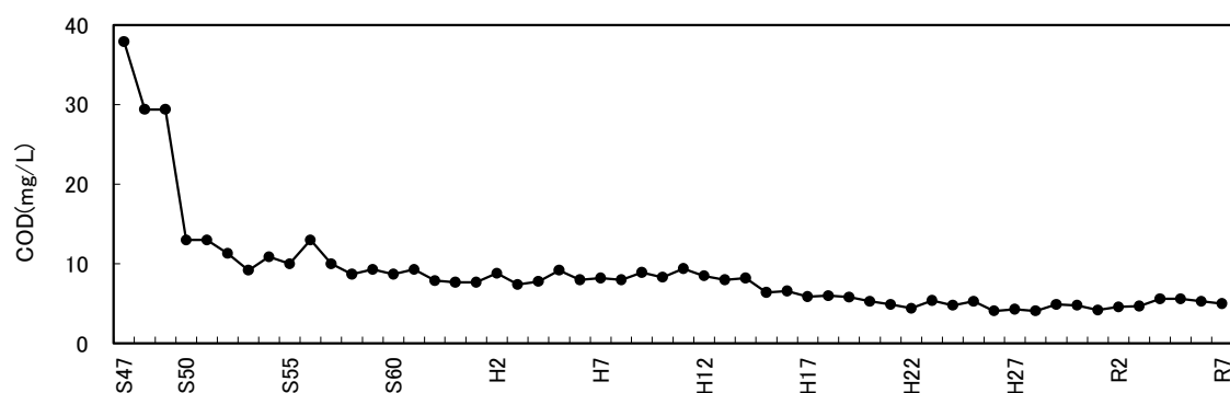
図7 山王川(所橋)のCODの推移
