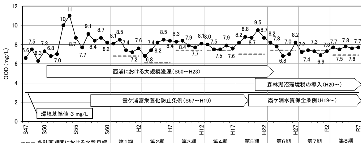
図 1 COD (全水域平均) の推移
