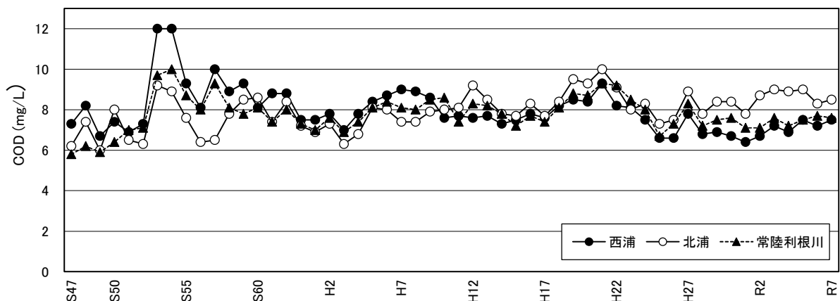
図 2 COD (水域別) の推移
