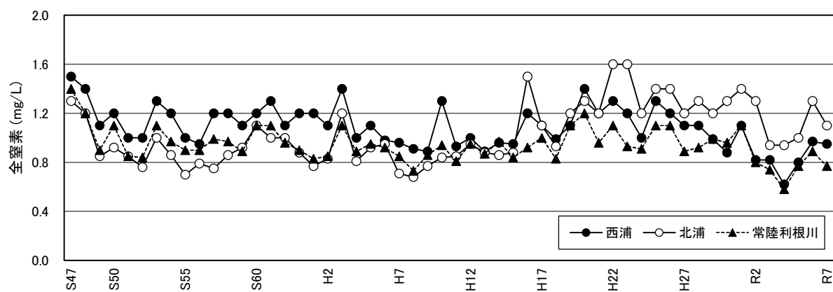
図4 全窒素(水域別)の推移
