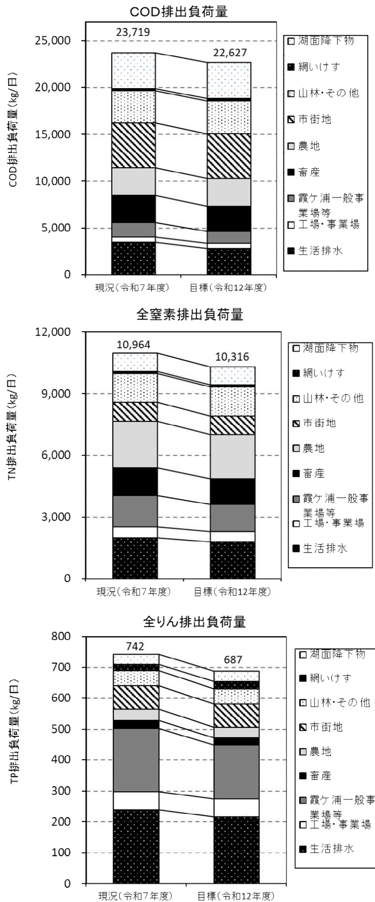
図 13 霞ヶ浦における排出負荷量（現況及び目標）
