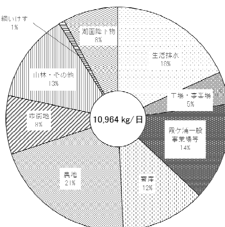
霞ヶ浦におけるTP排出負荷量(令和7年度)
