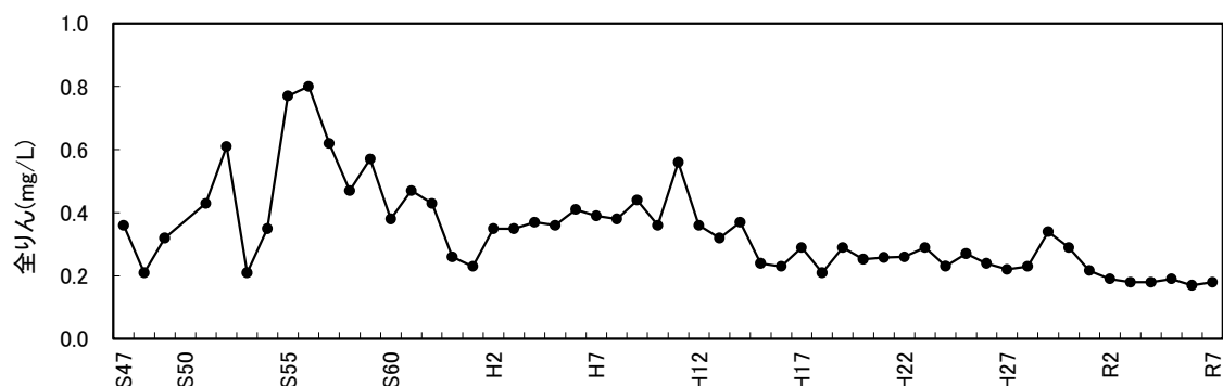
図9 山王川(所橋)の全りんの推移
