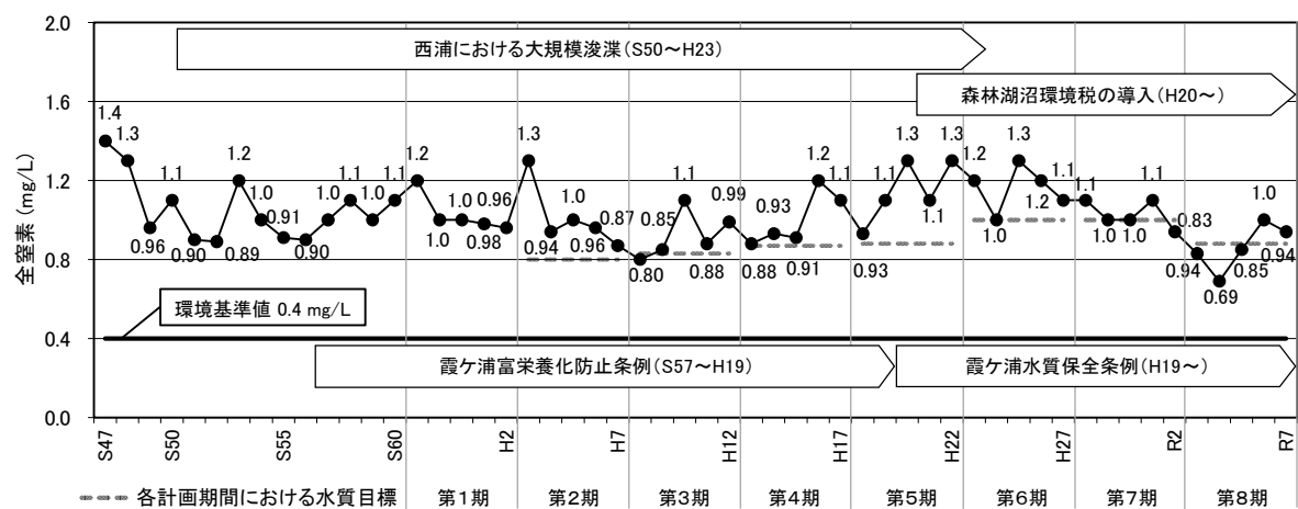
図3 全窒素(全水域平均)の推移
