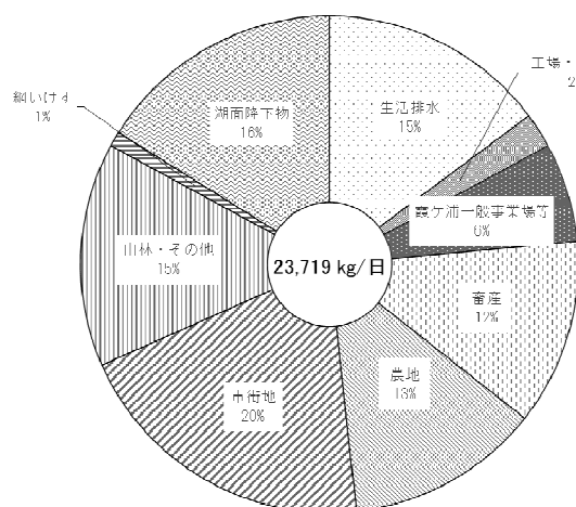
霞ヶ浦におけるTP排出負荷量(令和7年度)
