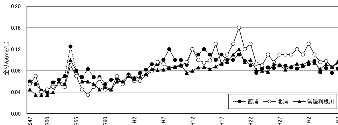
図6 全りん(水域別)の推移
