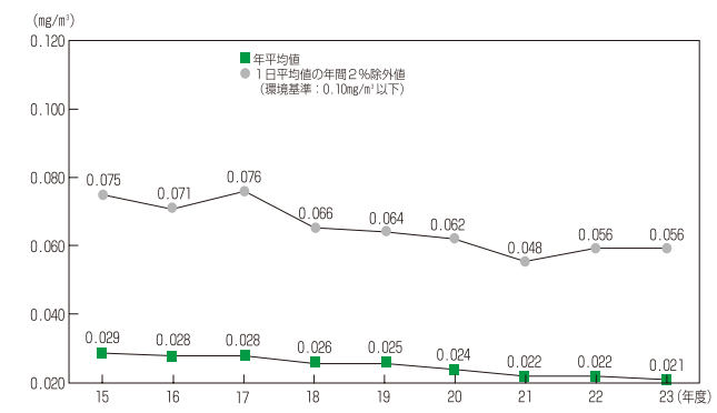
図表2-1-13 浮遊粒子状物質の年度別推移(自排局平均)
