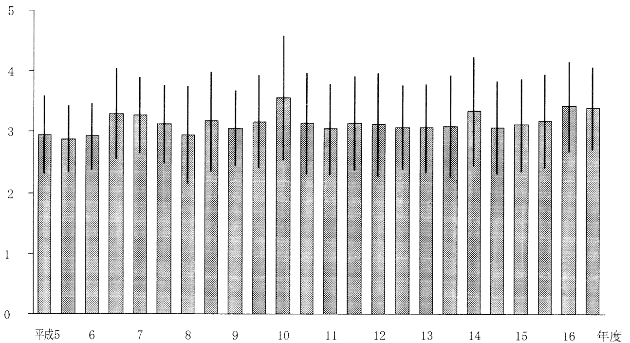
空間 \gamma 線量率（サーベイ）経年変化 【大洗地区】
