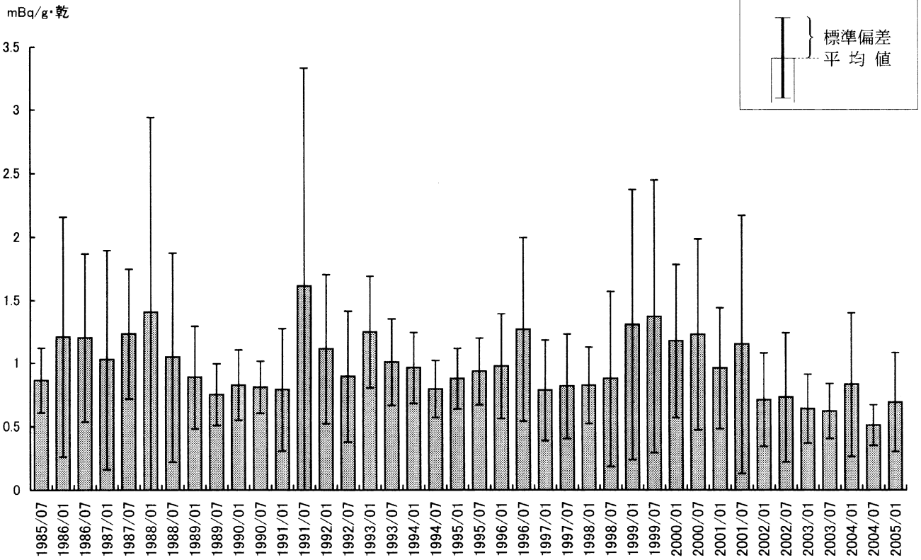
海底土中の 137 Cs濃度の経年変化（県測定分）
