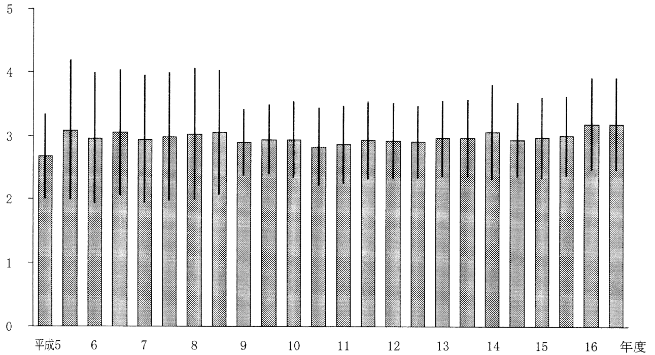
空間 \gamma 線量率（サーベイ）経年変化 【東海地区】
