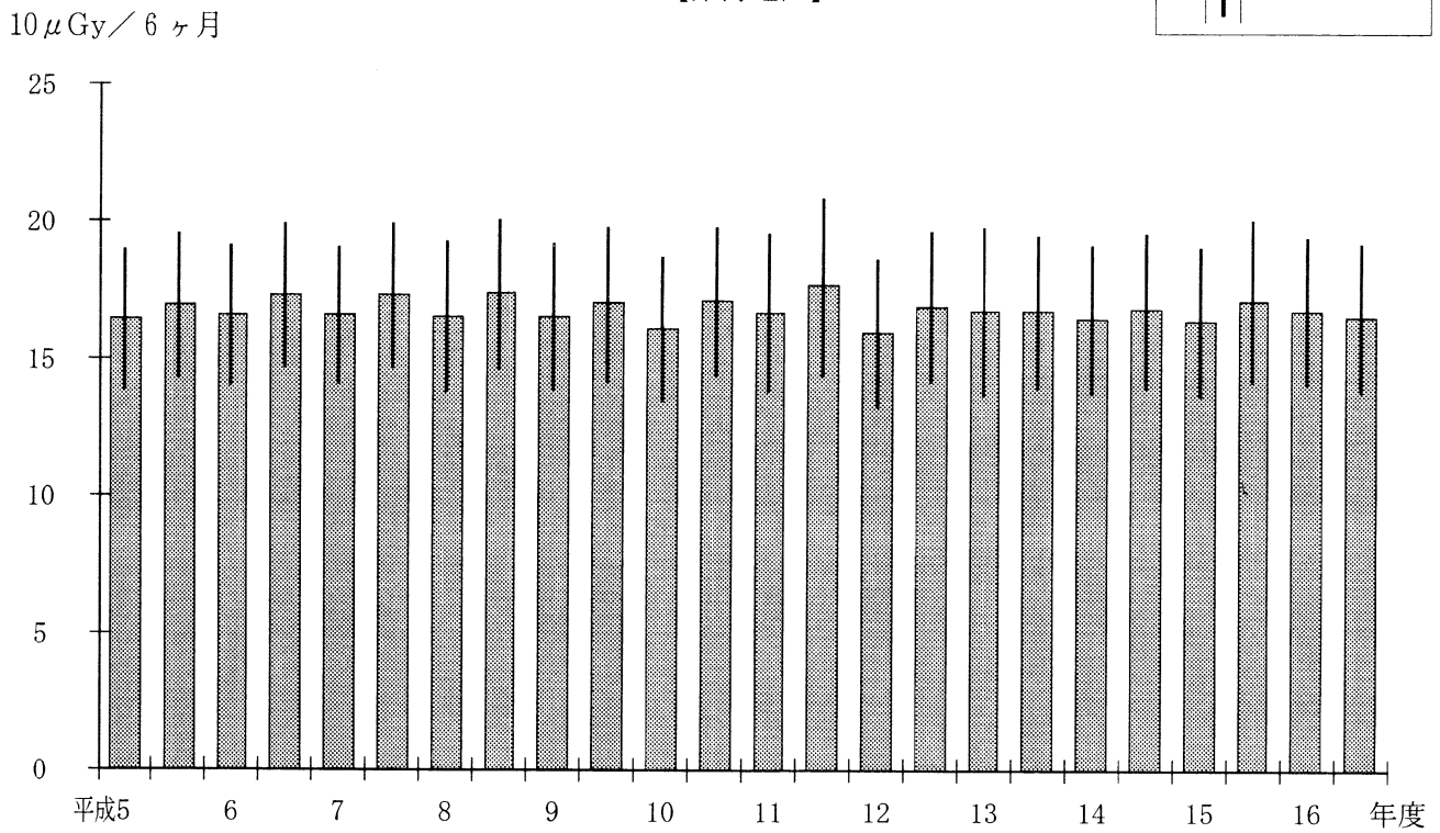
積算線量経年変化 【東海地区】
