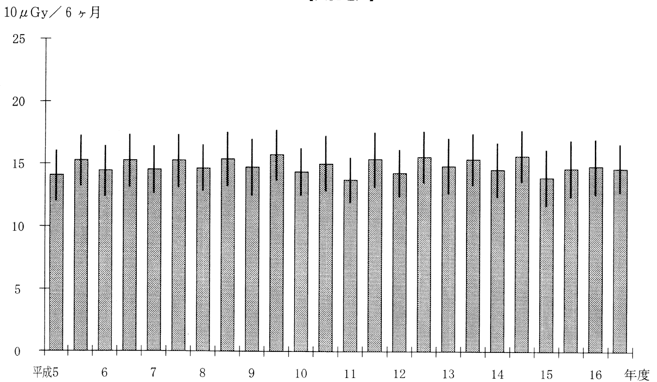
積算線量経年変化 【大洗地区】
