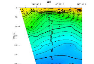
図5. 鉛直水温
