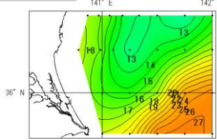
図2. 水深別水温
