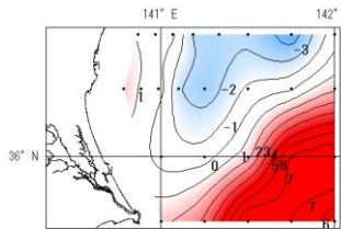
図4. 水深別水温平年差
