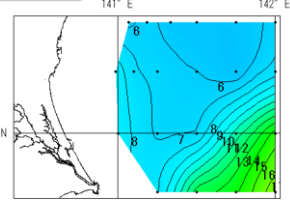
図1. 海況の現況 (9月3日)
