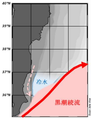
図1. 海況の現況 (9月3日)
