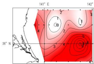
図3. 水深別水温前月差
