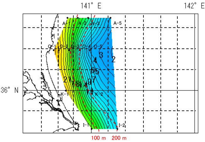
図8. 令和8年9月の底水温(*海底直上約5～20m)
