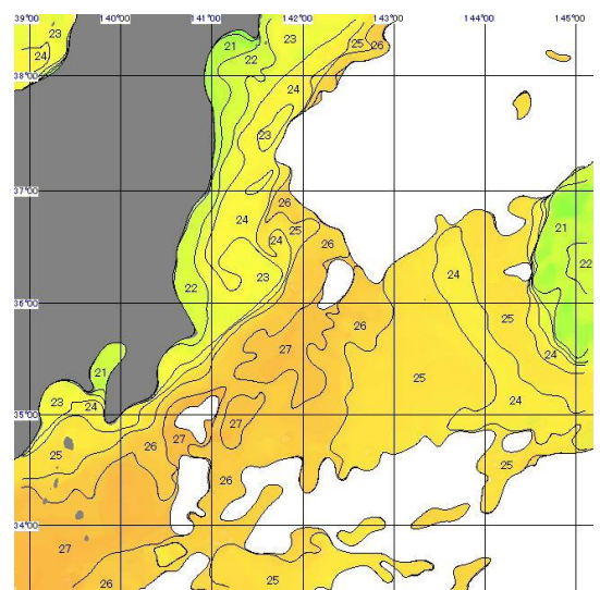
図2. 10月23日の人工衛星NOAA海面水温図.
