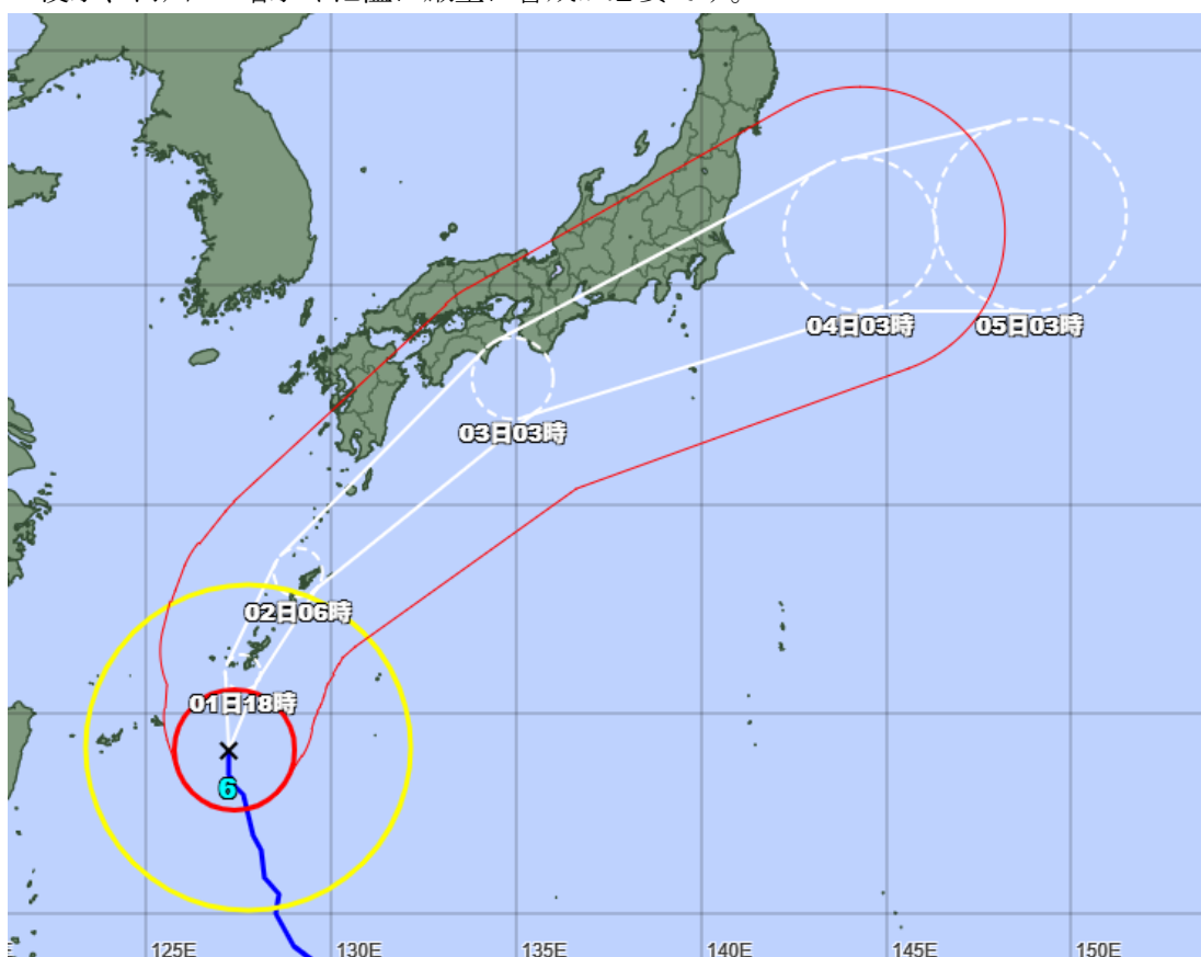
2026年6月1日8時 進路予報図
