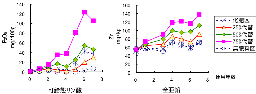
図2 豚ふん代替区における土壌成分の年次変化
