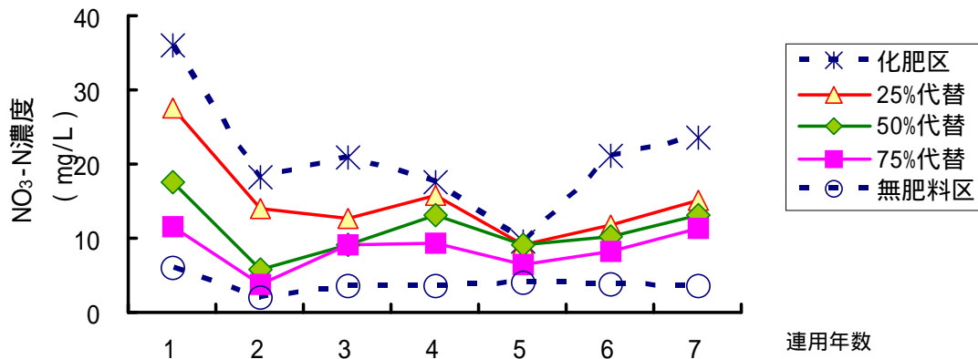
図1 豚ふん代替区における浸透水の年平均硝酸態窒素濃度の年次変化 年平均硝酸態窒素濃度：年間の硝酸態窒素溶脱量 / 年間の浸透水量
