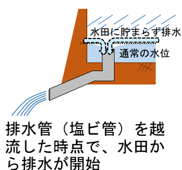
田んぼダム用の落水柵
