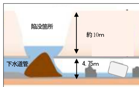
陥没箇所の横断面図（イメージ）
