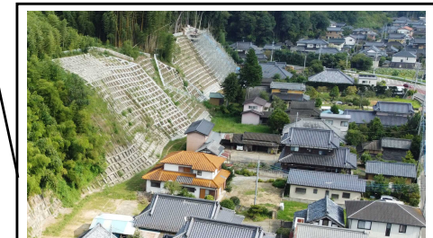
法面对策: 弁才天2地区(小美玉市)
