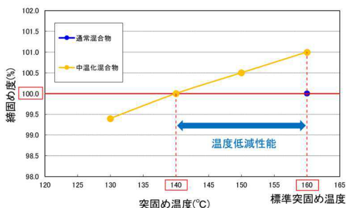
図3-2-6 温度—突固め度のグラフ（作成例）
