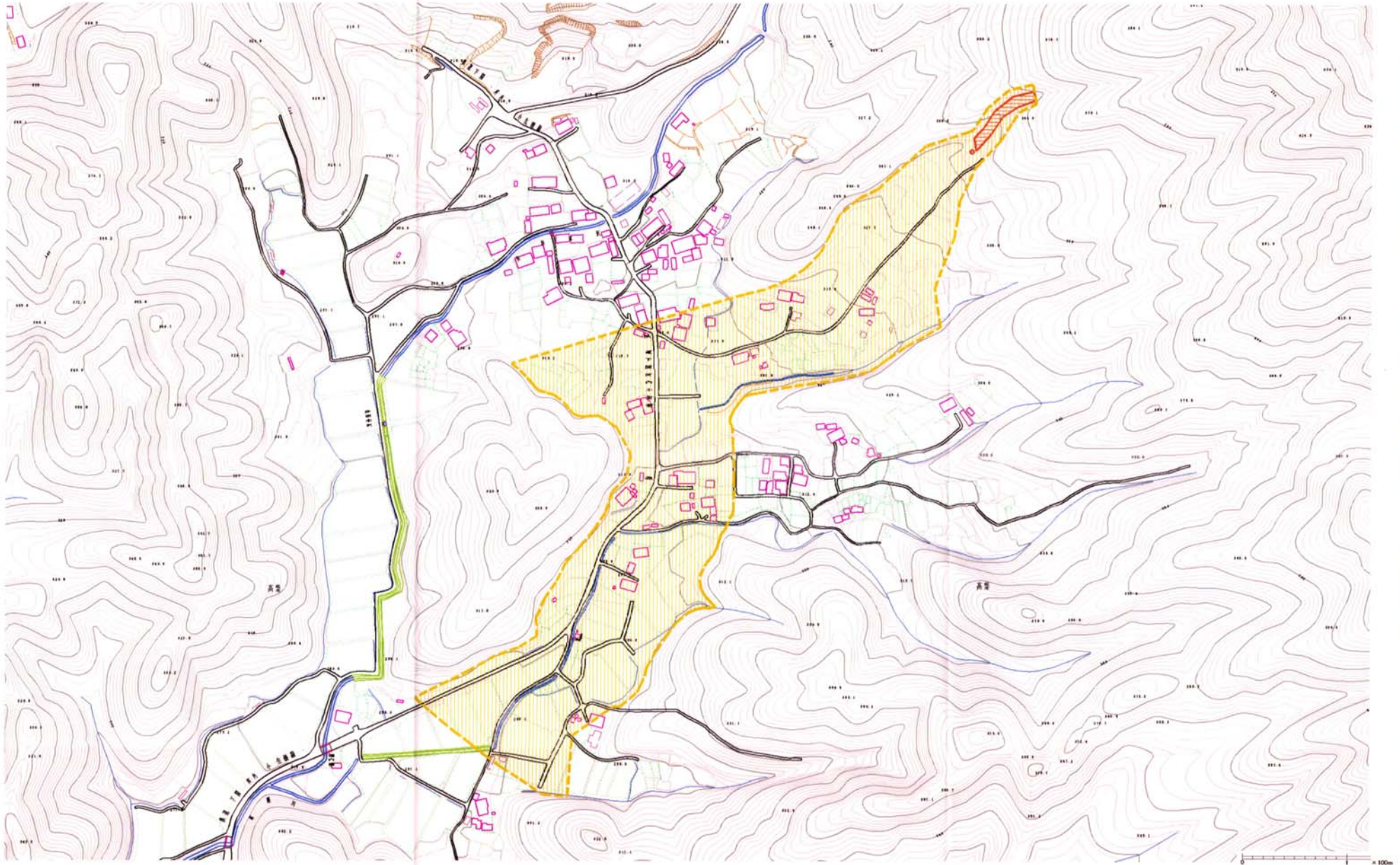
様式-2（土） 土砂災害警戒区域・土砂災害特別警戒区域 区分図（その1）
