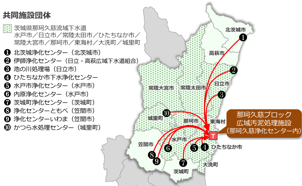
図 V-8 那珂久慈ブロック広域汚泥処理の概要
